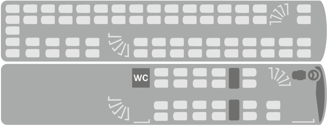
Variante 1 S 431 DT - 3 étoiles - 85 places assises + WC
